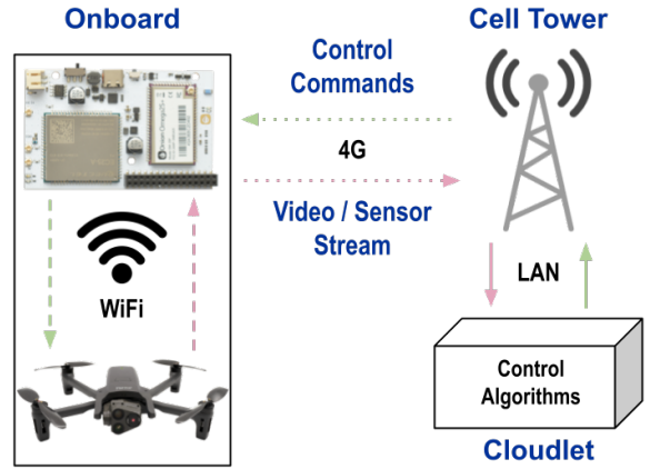
Fig. 1: Edge Offload Pipeline
