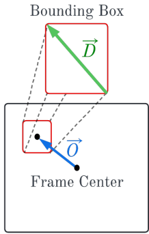
Fig. 23: \vec{O} & \vec{D}
